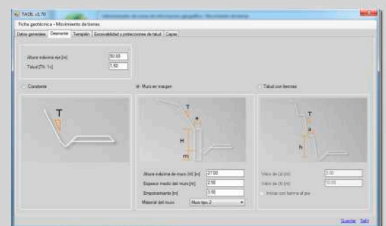
Ejemplo módulo TDB SIG. Geotécnia
